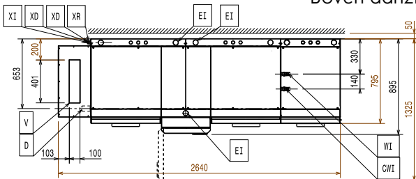
Boven aanzicht
