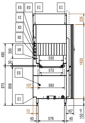
Zij aanzicht
